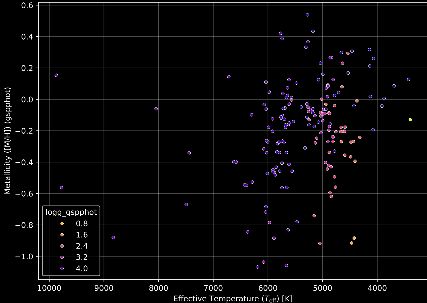
APOGEE DR17 Field: [271-34-O_TESS] Stellar Population Parameters (n= 177)
